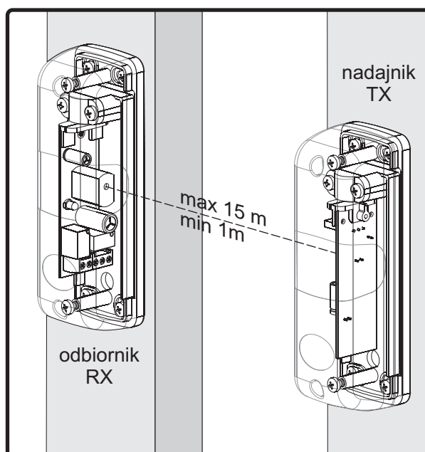
Rys. 1 Przykładowe umiejscowienie nadajnika względem odbiornika
