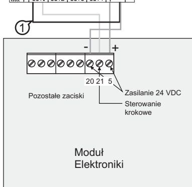
Schemat 3. Przykład połączenia sterownika napędu bramy Hormann z odbiornikiem Rival434.
