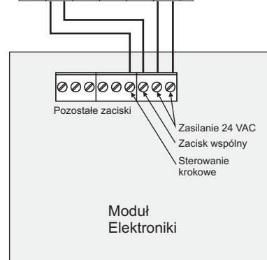
Schemat 4. Przykład połączenia sterownika napędu bramy NICE z odbiornikiem Rival434.
