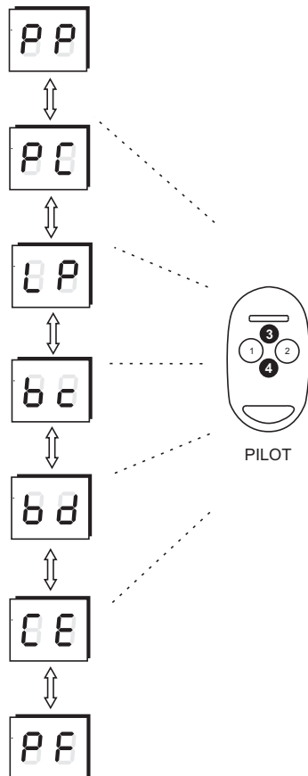
Rys.6. Opcje menu głównego Pojawiające się po zadeklarowaniu PILOTA
