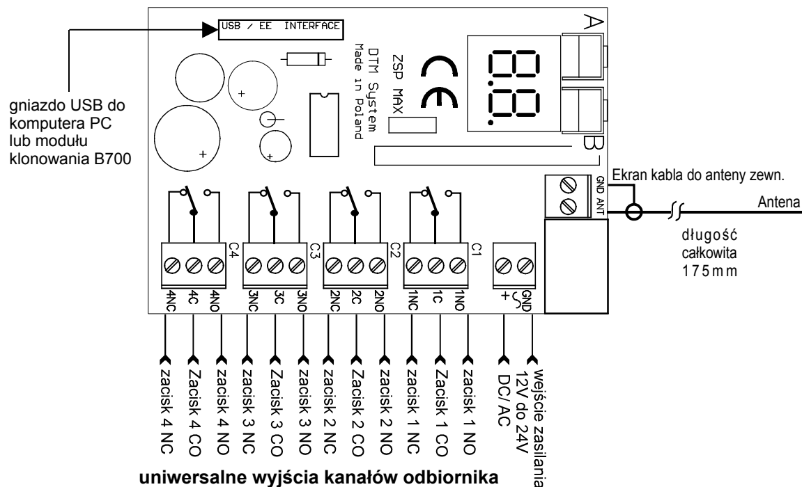
rys 1. Schemat elektryczny instalacji odbiornika MAX
