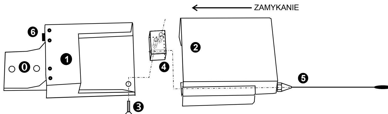
rys.3 Widok obudowy odbiornika MAX oraz elementów do montażu anteny
