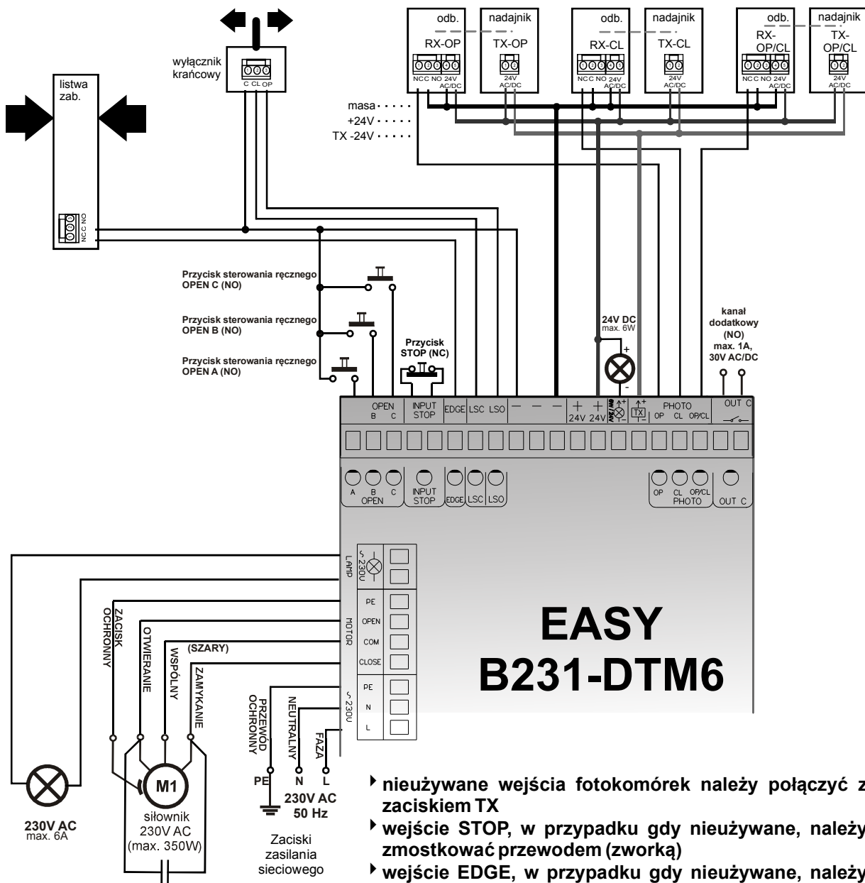
Rysunek 2. Sposób podłączenia zacisków sterownika EASY B231-DTM6
